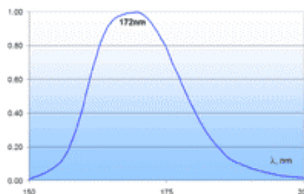
発光特性
